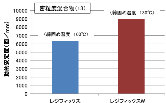
図-2 動的安定度の比較 (例)
