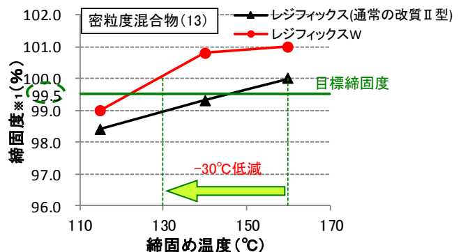
図-1 マーシャル締固め温度と締固め度の関係 (例)
