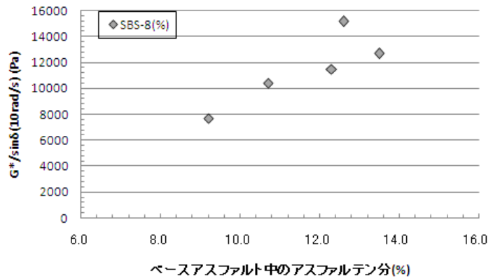
図-4.ベースアスファルト（針入度 60/80）のアスファルテン分と PMA の DSR 特性 (G*/sinδ) の関係
